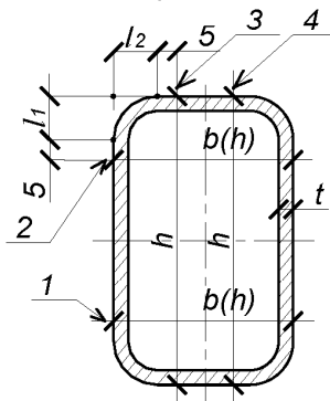
Рисунок 3 – Схема измерения размеров квадратных и прямоугольных профилей
